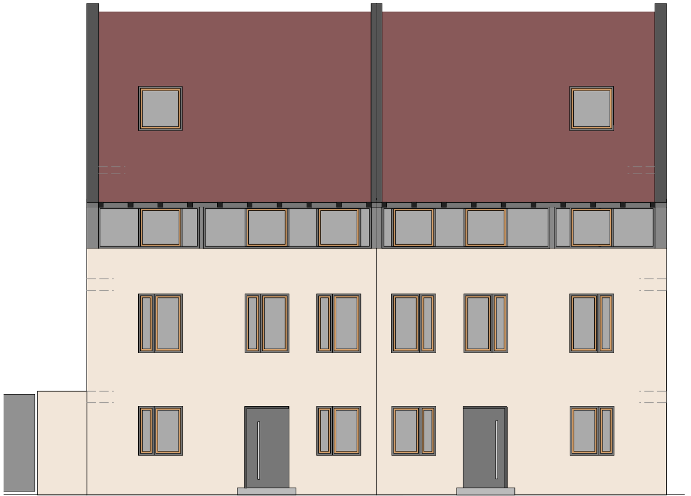
ANSICHT NORD-WEST
