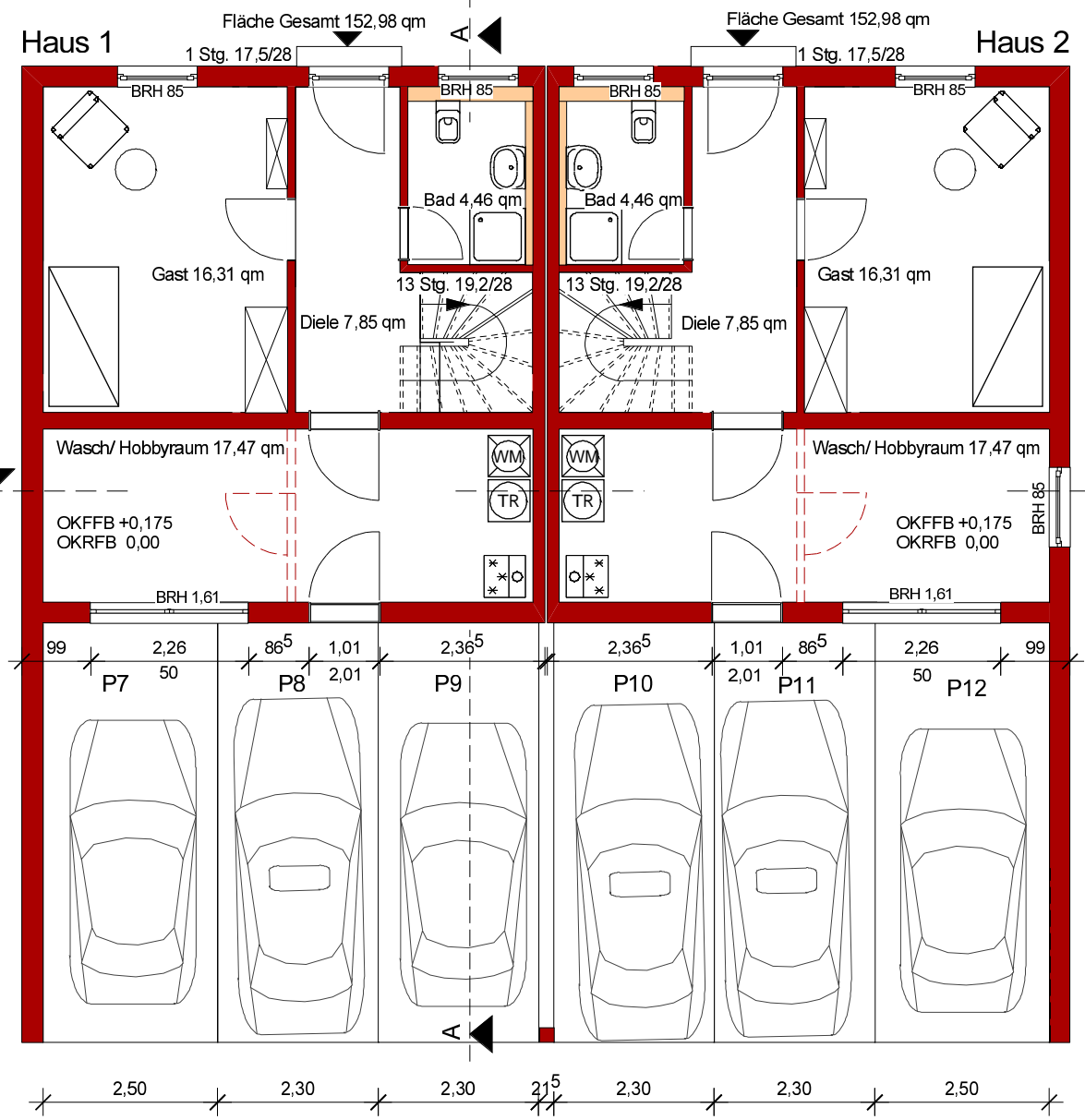
ERDGESCHOSS
